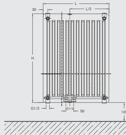
Achteraanzicht Type 20/21/22
