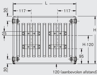
Achteraanzicht Type 10/11
