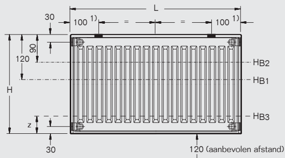
Achteraanzicht Type 20/21/22/30/33
