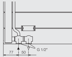
2 pijps - onderaan
