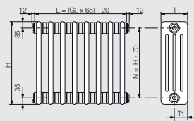
2-pijps, zijkant
