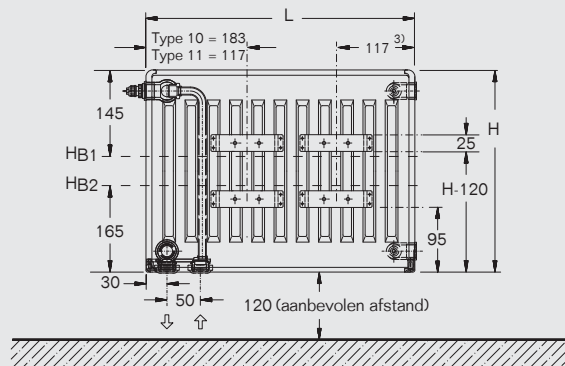
Achteraanzicht type 10/11
