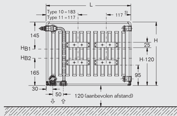
Achteraanzicht type 10/11
