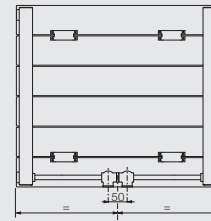
2 pijps - middenaansluiting
