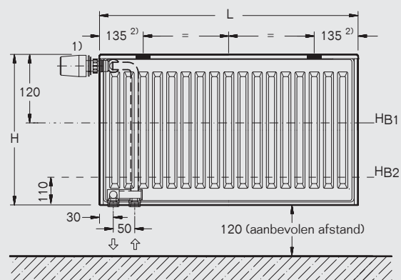
Achteraanzicht type 20/21/22/30/33
