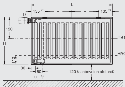
Achteraanzicht type 20/21/22/30/33
