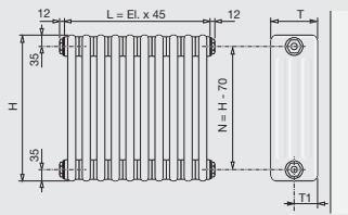
2-pijps, zijkant
