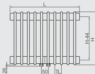
2 pijps - middenaansluiting
